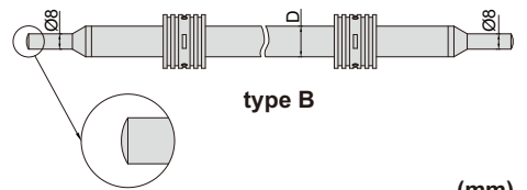
6310-300
